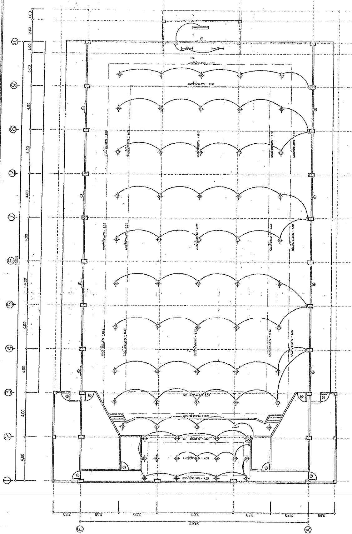
แบบแปลนระบบแสงสว่าง ขนาดจริง
