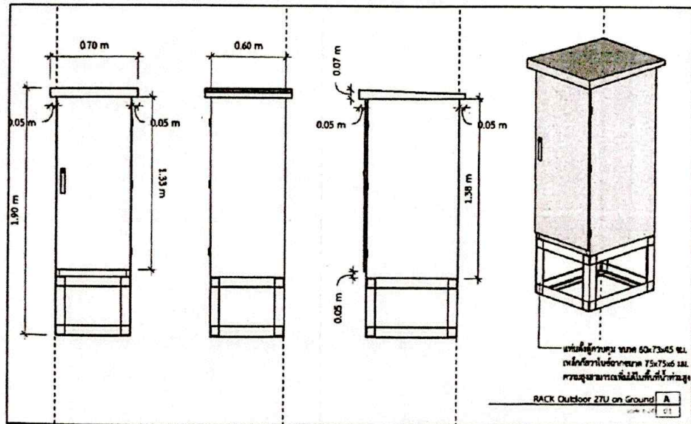
แบบตู้เก็บอุปกรณ์ (Rack)
