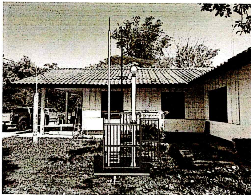
ภาพถ่ายสถานที่ที่จะติดตั้งสถานีรับสัญญาณดาวเทียมอ้างอิง CORS (ถ่ายภาพจากทิศตะวันตกไปทิศตะวันออก)
