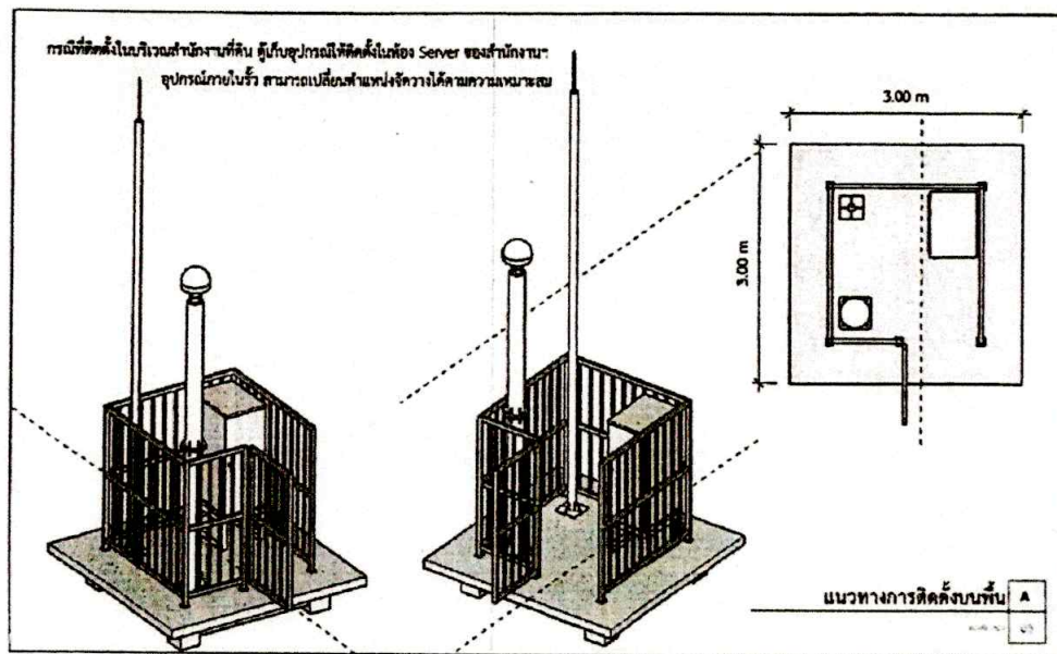
แบบในการติดตั้งสถานีรับสัญญาณดาวเทียม แบบบนพื้นดิน
